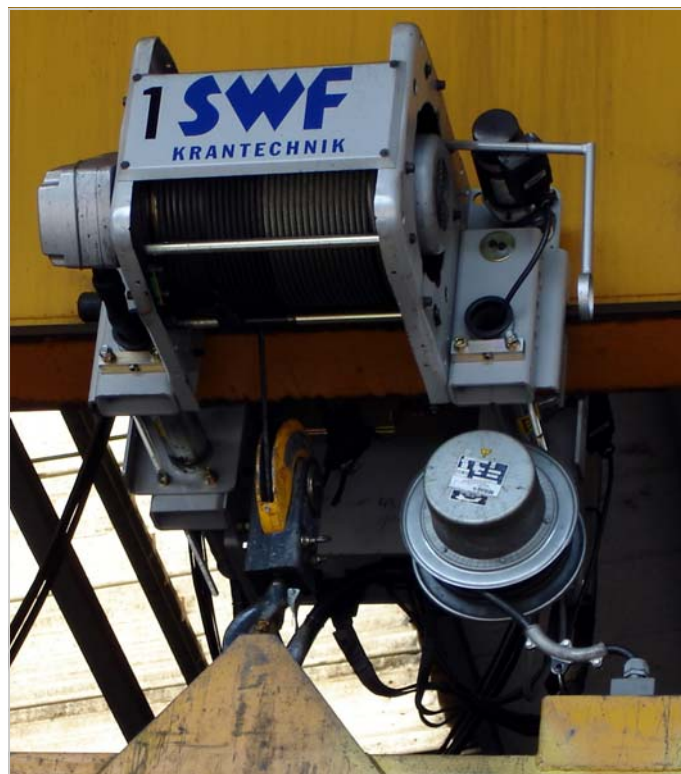
Federleitungstrommel für Magnetansteuerung wirtschaftliche Lösung für die Versorgung von einem Magnethebergerät
