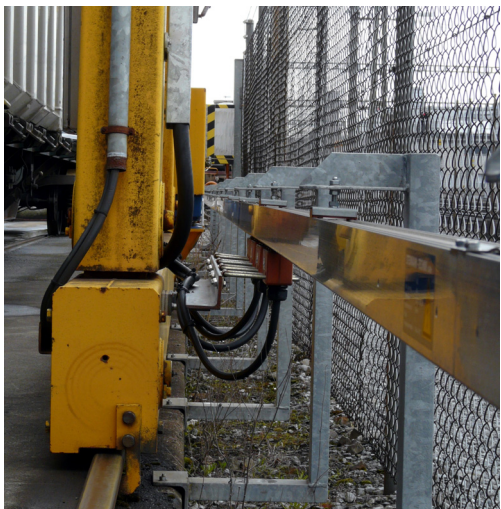
Stromabnehmerwagen 4 Einheiten parallel mit Mitnehmer-Gabel
