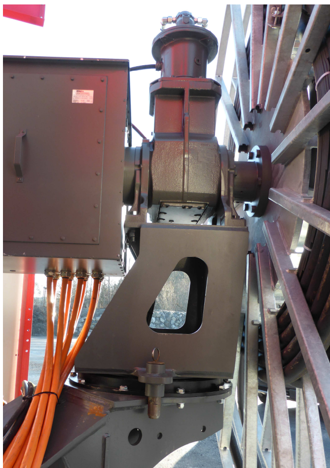
Ansicht Hydraulikmotorantrieb, mit Schleifringbox ausgestattet mit 3+PE, 1000A, mit drehbarer Halterung für die exakte Ausrichtung der Trommel
